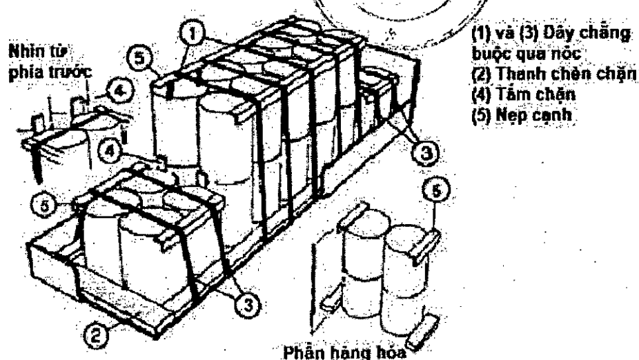
Hình 4.2. Minh họa mô tả cách xếp các cuộn giấy không đồng đều về chiều cao
