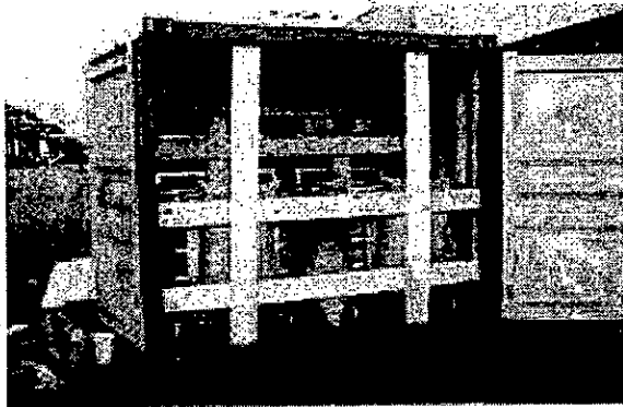
Hình 5.2. Minh họa về các thùng hàng tải trọng trung bình được chồng đôi trong công te nơ
